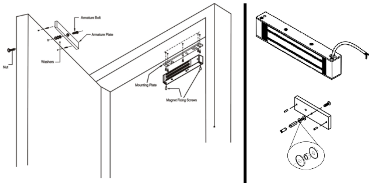
Рис. 1. Схема кріплення пристрою
